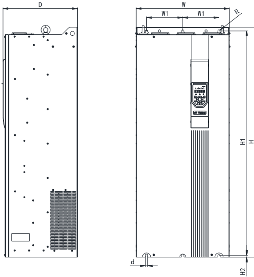
560kW~900kW 壁挂式安装示意图
