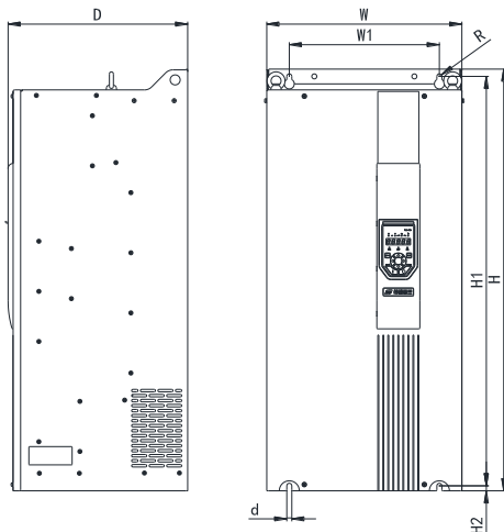
160kW~500kW 壁挂式安装示意图
