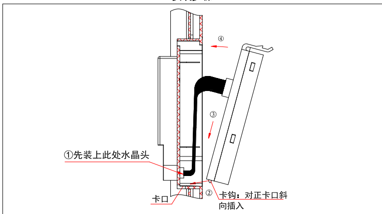
图 3-7 各机型手操盒的拆卸与安装步骤
