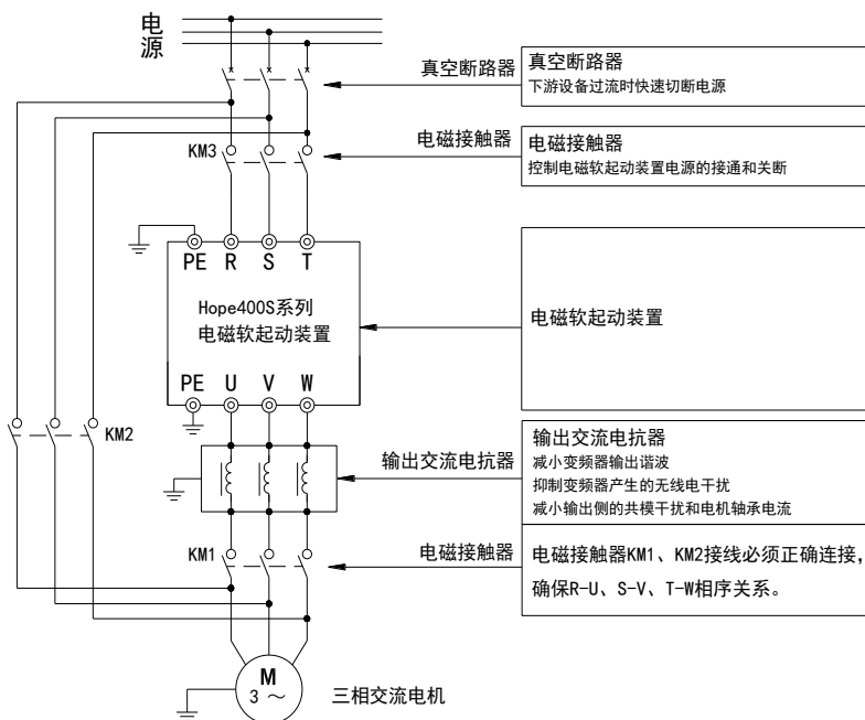
图3-9 Hope400系列电磁软起系统连接示意图
