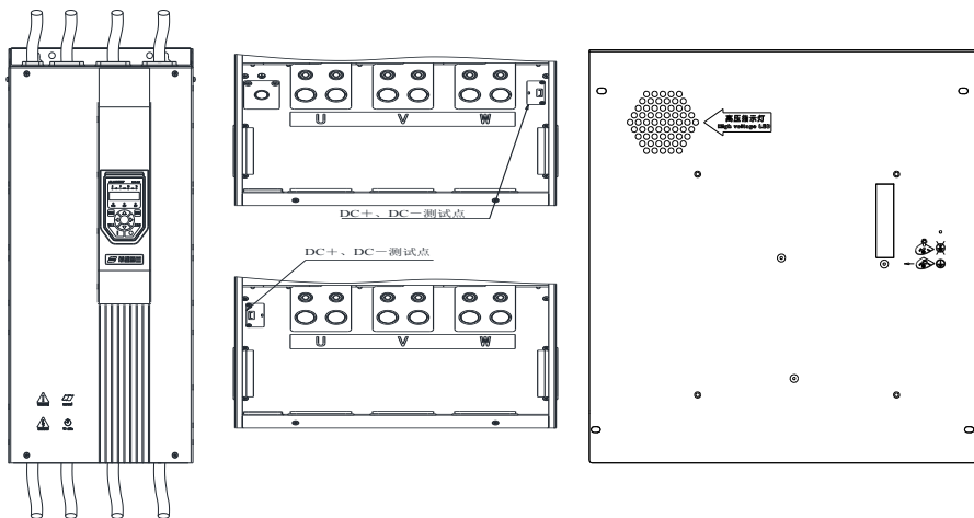
整机接线效果图
