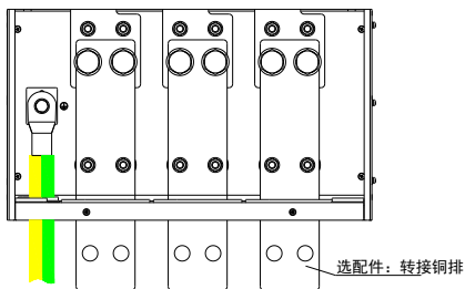
Hope400S560T4~Hope400S900T4系列软起装置 转接铜排安装示意图
